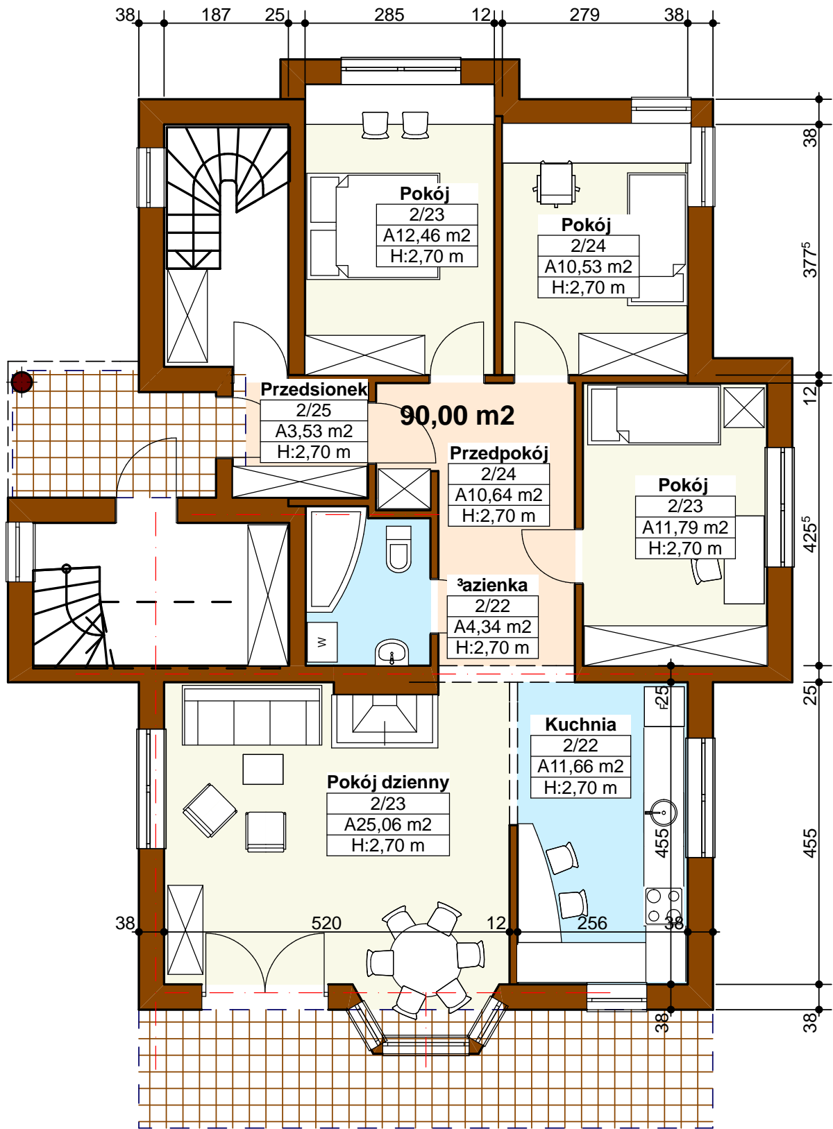
RZUT PARTERU
