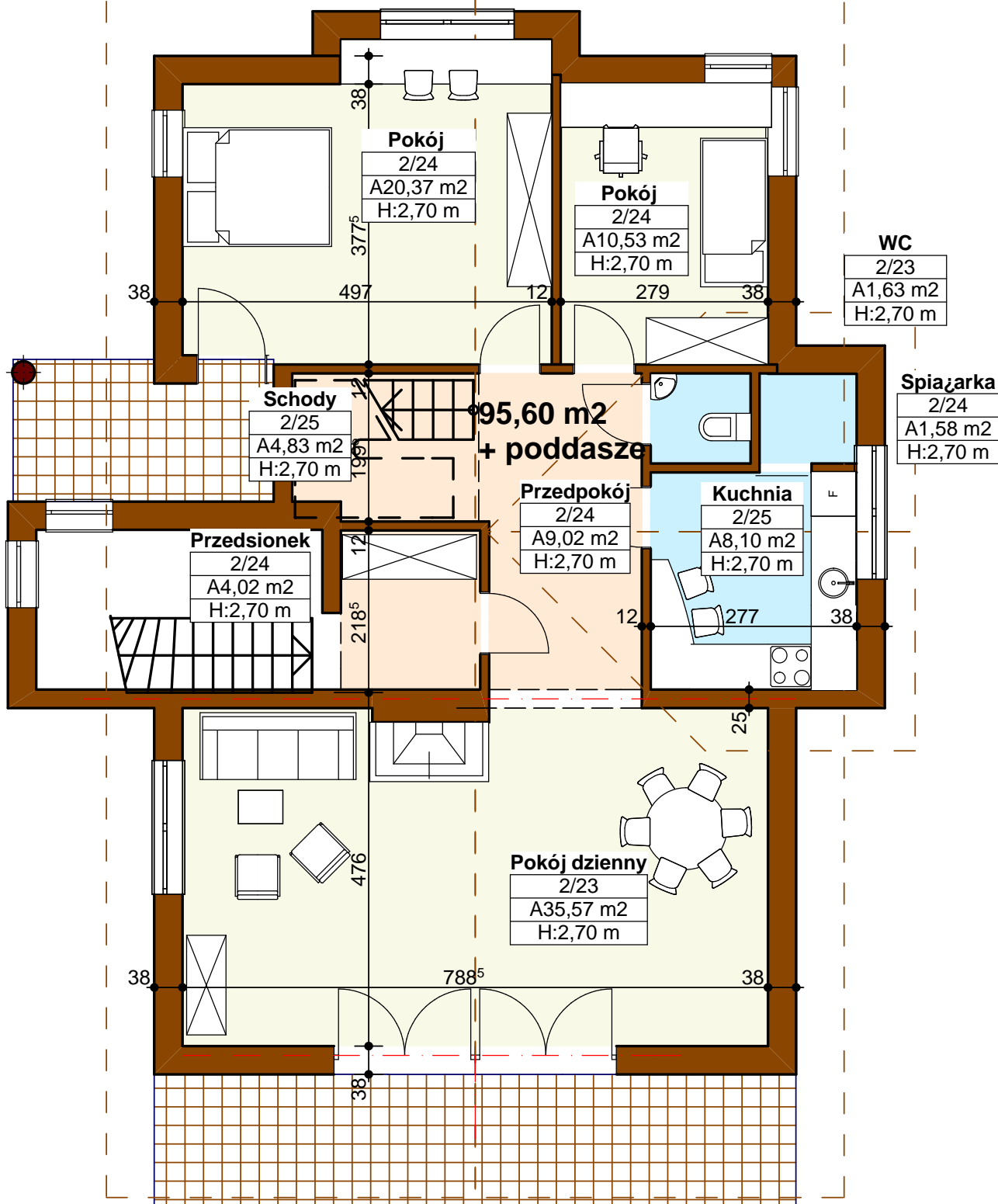
RZUT PIĘTRA
