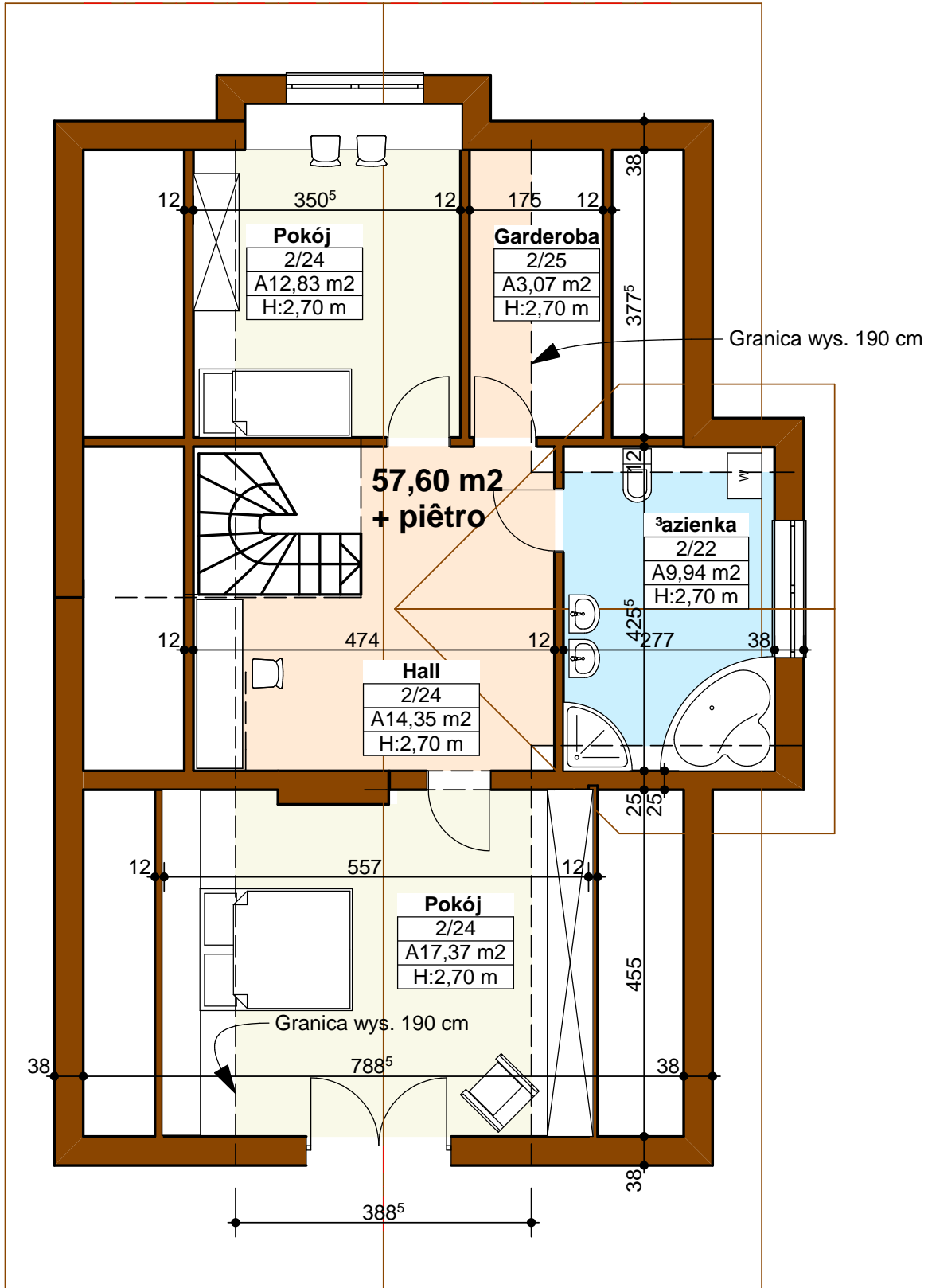
RZUT PODDASZA
